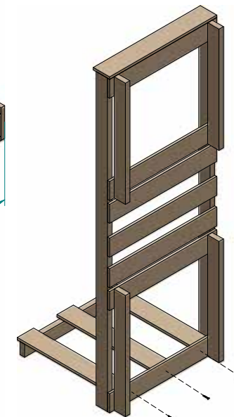
Boční palety pro dopravu v horizontální poloze
